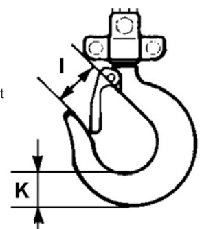
Abb. 4 Lastenhaken
