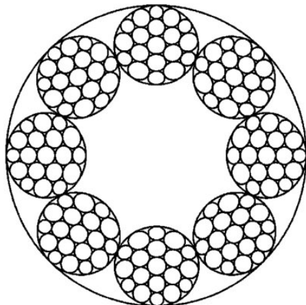
Aufzugseil
