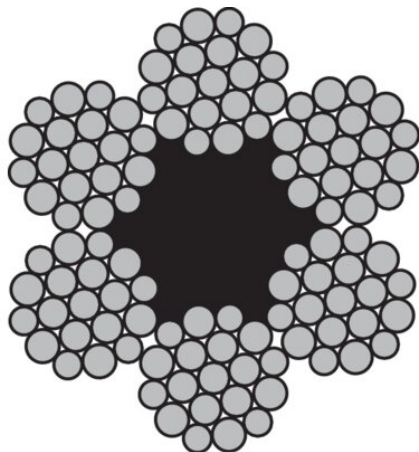
Aufzugseil
